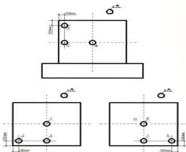
Рисунок 19 – Схема расположения термометров в железобетонных конструкциях
