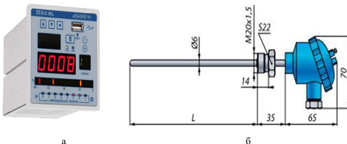
Рисунок 5 – Восьмиканальный микропроцессорный прибор ТМ 5103 (а) и термометры сопротивления ТМ-1288/1 (б)
