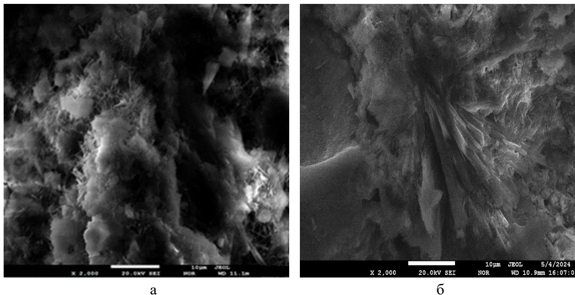
а – образование начальных кристаллов; б – слоистых пакетов портландита, X 2000
