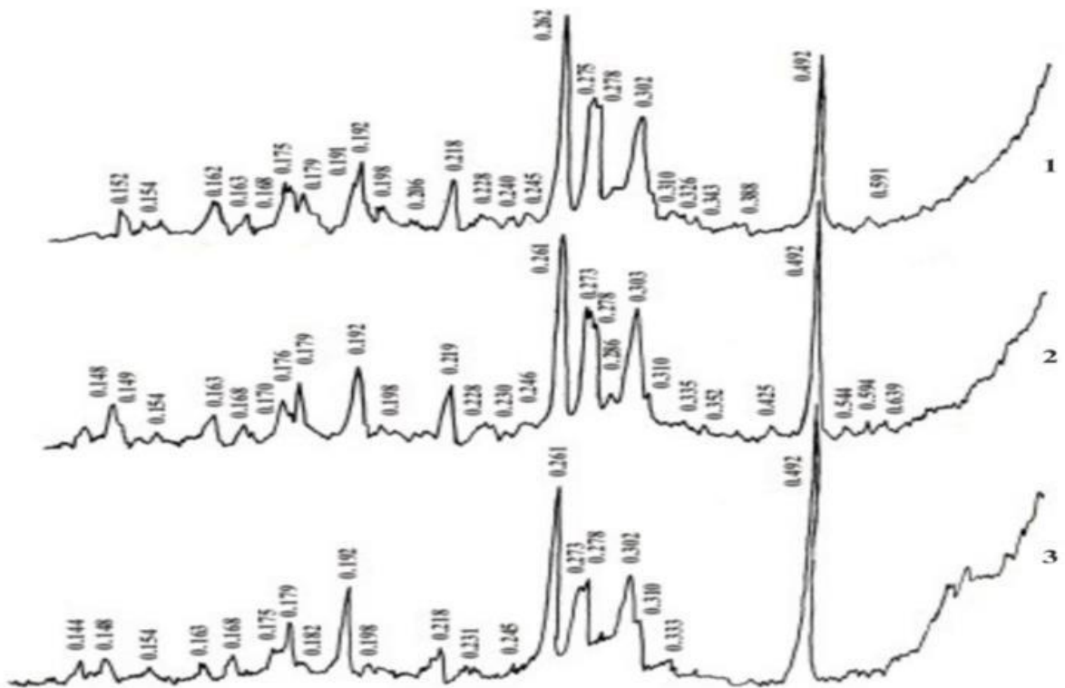
Рисунок 11 – Рентгенограммы C3S в возрасте 28 суток нормального твердения: без добавки (1), с добавкой 20% отходов обогащения Балхашского ГОК (2) и 20% отходов обогащения Балхашского ГОК и микрокремнезёма
